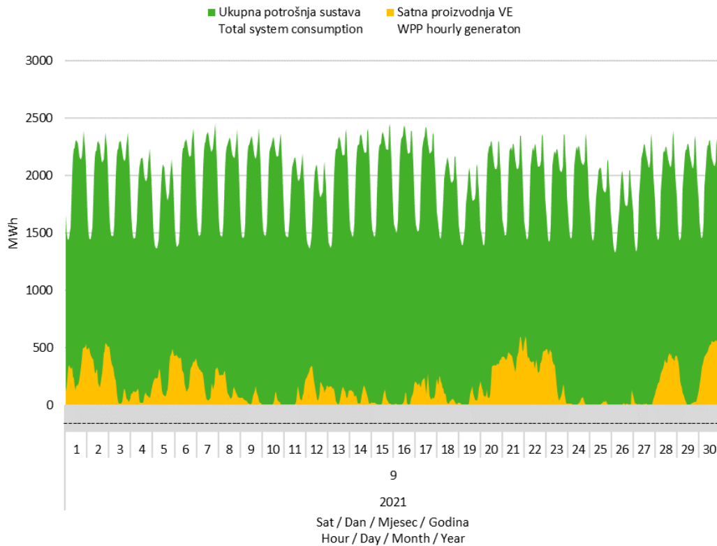
Slika 7 Usporedba satnog dijagrama opterećenja sustava i proizvodnje vjetroelektrana u rujnu 2021. godine
