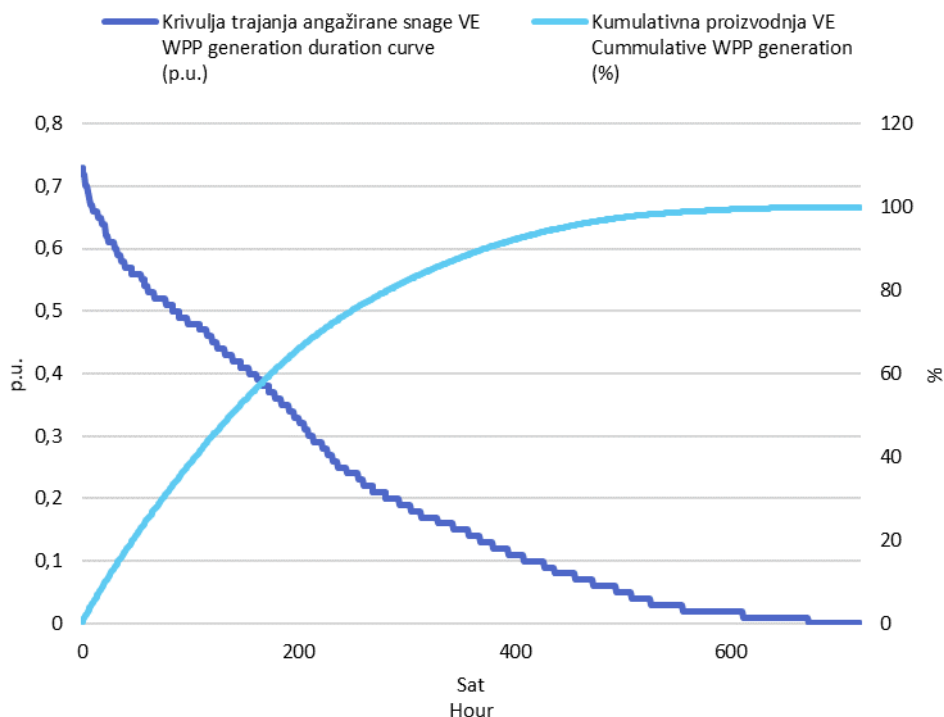
Slika 3 Krivulja trajanja angažirane snage svih VE i kumulativna proizvodnja VE u rujnu 2021. godine u jediničnim vrijednostima
