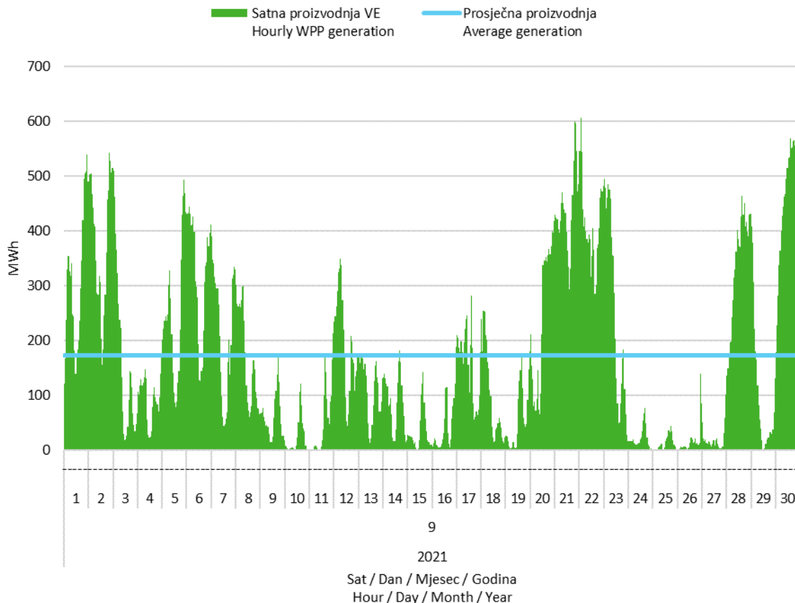
Slika 2 Satna proizvodnja svih vjetroelektrana u rujnu 2021. godine
