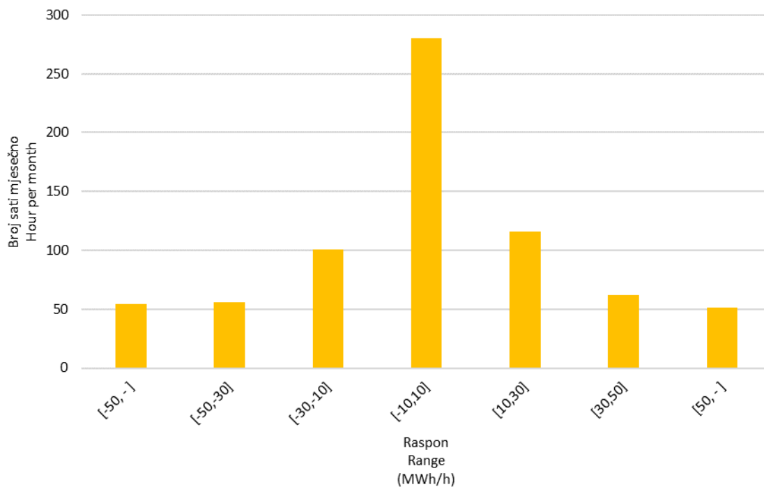
Slika 10 Statistička raspodjela satnih promjena proizvodnje VE u rujnu 2021. godine Figure 10 Statistical distribution of WPP hourly output variations in September 2021
