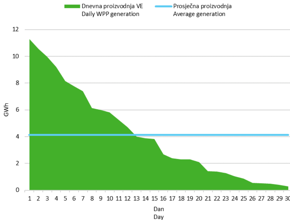
Slika 6 Krivulja trajanja dnevne proizvodnje vjetroelektrana u rujnu 2021. godine
