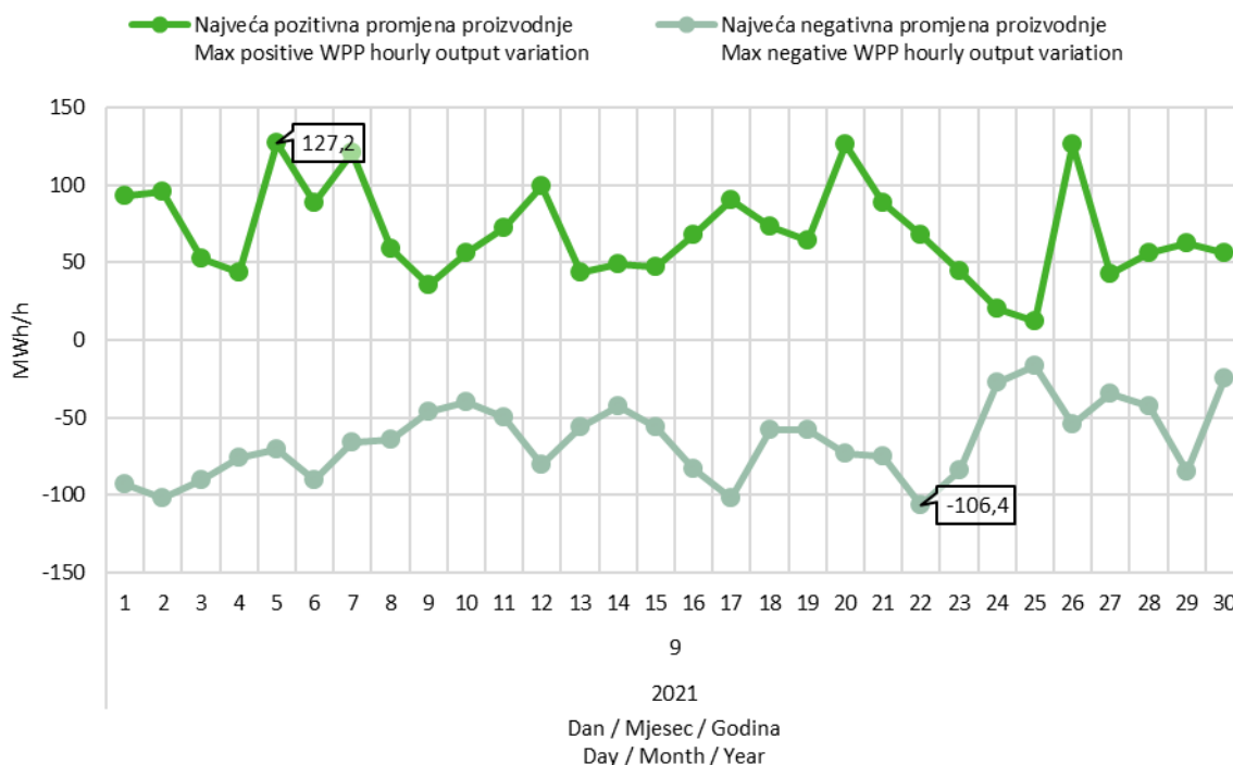
Slika 9 Maksimalna pozitivna i maksimalna negativna promjena satne proizvodnje VE u rujnu 2021. godine
