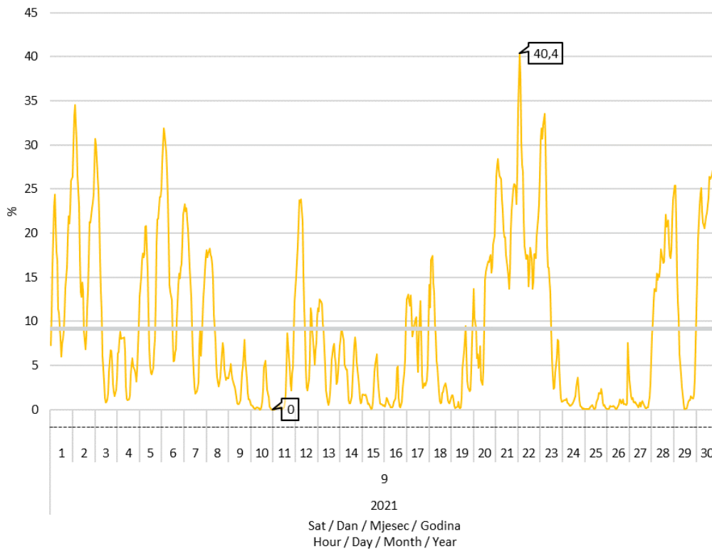
Slika 8 Udio proizvodnje vjetroelektrana u pokrivanju satnog opterećenja elektroenergetskog sustava u rujnu 2021. godine
