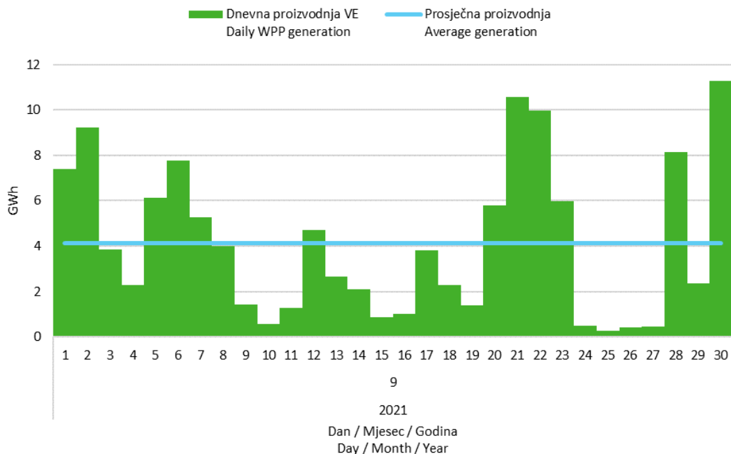
Slika 5 Dnevna proizvodnja svih vjetroelektrana u rujnu 2021. godine
